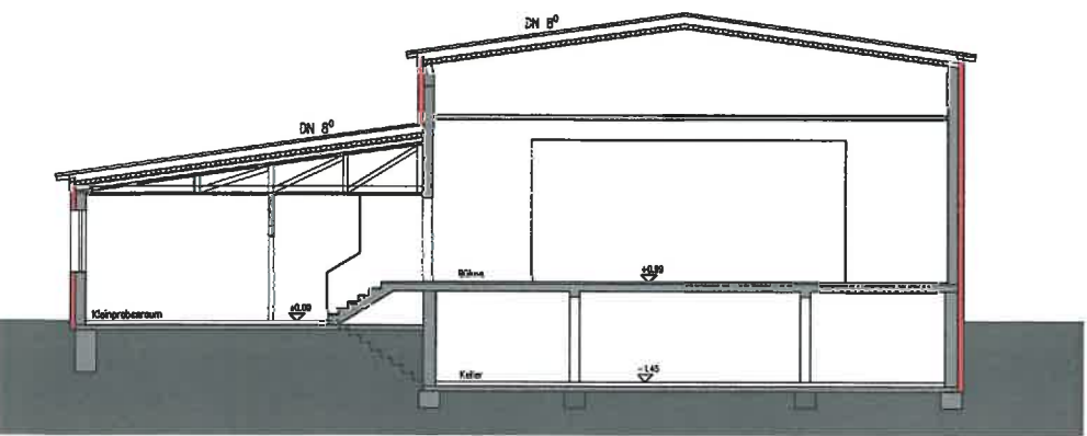
Schnitt Bühne
