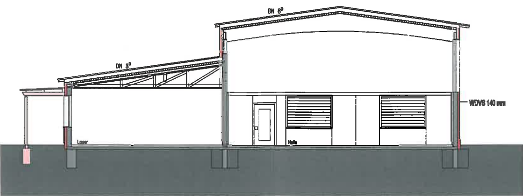
Schnitt Lagerhalle
