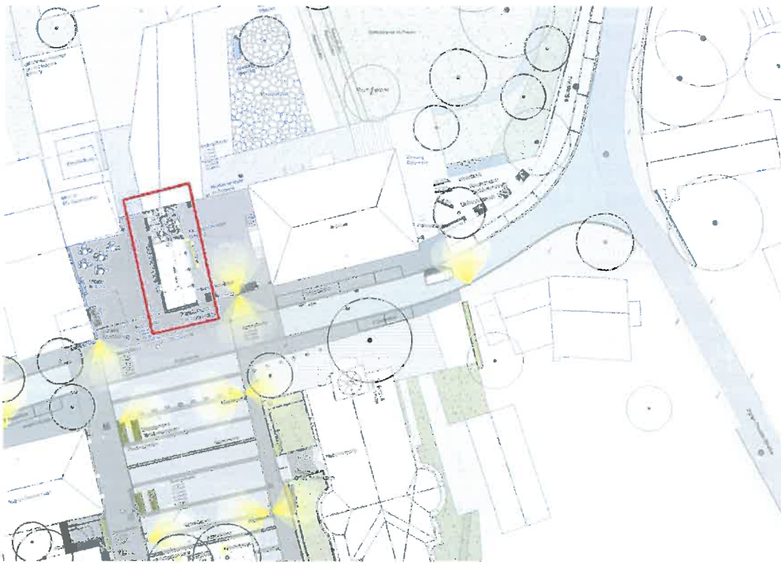
Abb. 1: Grundriss der Toiletten in der Garage vor der Remise
