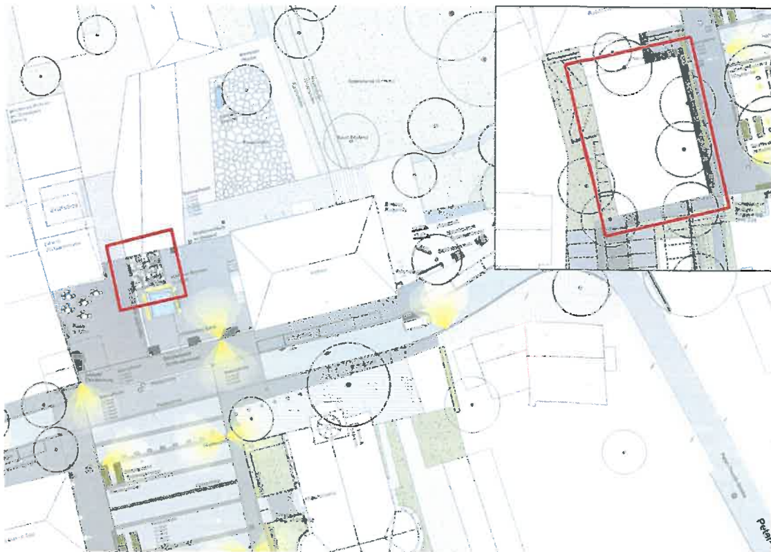
Abb. 3: Lageplan Standort auf Platz bei Abriss der Garagen bis zum Bau des Vereinshauses
